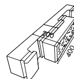
Färdig dubbelsidig murbredd 200 mm. Ca 426 kg/m 2
