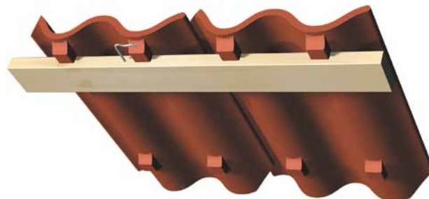
Bild 2: Monteringsvisning av takpannekrok
