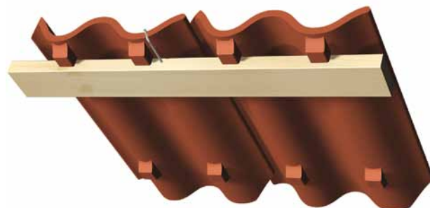
Bild 3: Alternativ till montering av takpannekrok
