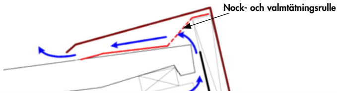
Bild 2: Montage vid Piano pulttak. Sörj för god ventilation vid denna montering.
