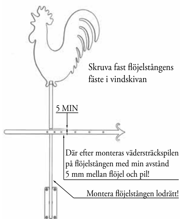
Montering av Vindflöjel
