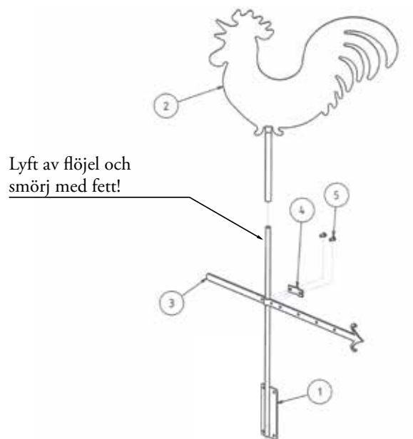
Underhåll vid uppstart av Vindflöjel
