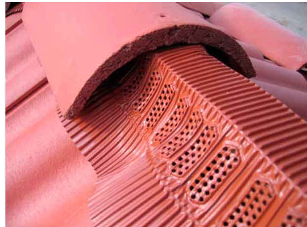
Kuva 6. Aseta harjatiili paikoilleen ja kiinnitä se sopivilla kiinnitysvälineillä. Tuotenumero 094391 tai 1147..
