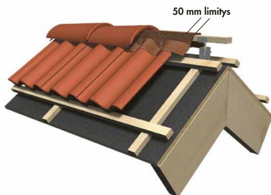
Kuva 2. Auma- ja harjatiivistenauha asennettuna.
