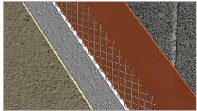
1. Putsuppbyggnad putsskikt 15-20 mm
