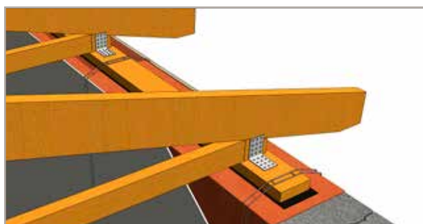
Bild 3.5 Vindförankring
