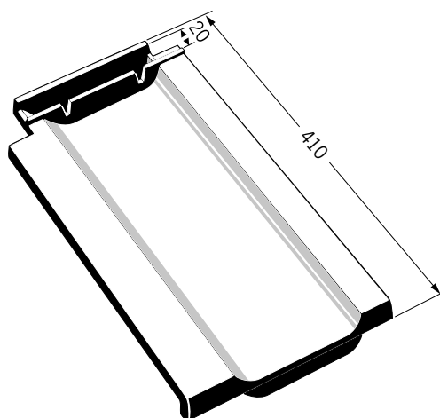
Dacapo Doppelwulstziegel
