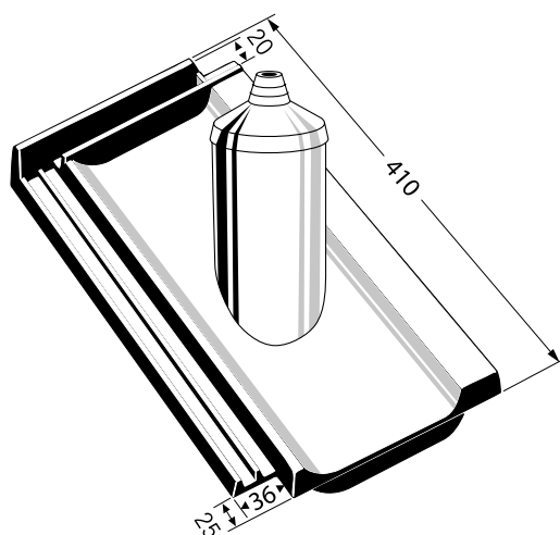
Dacapo Antennenziegel
