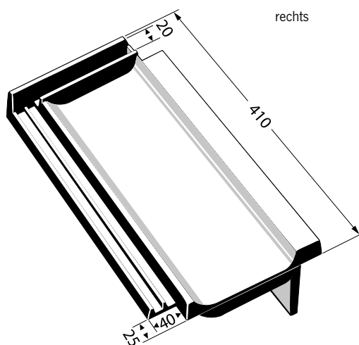
Dacapo Ortgangziegel
