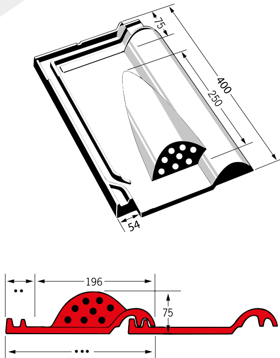
Garant Entlüftungsziegel
