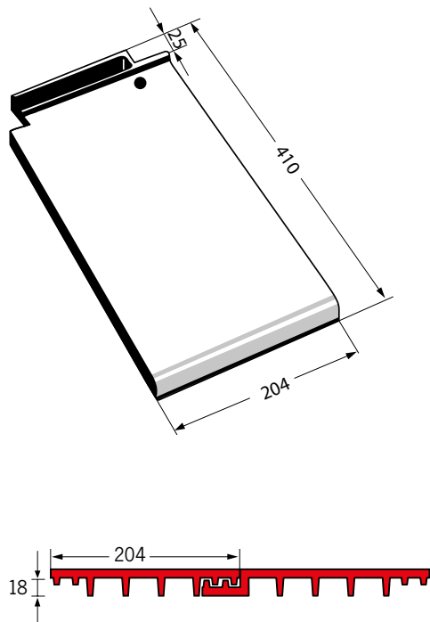
Piano Doppelwulst
