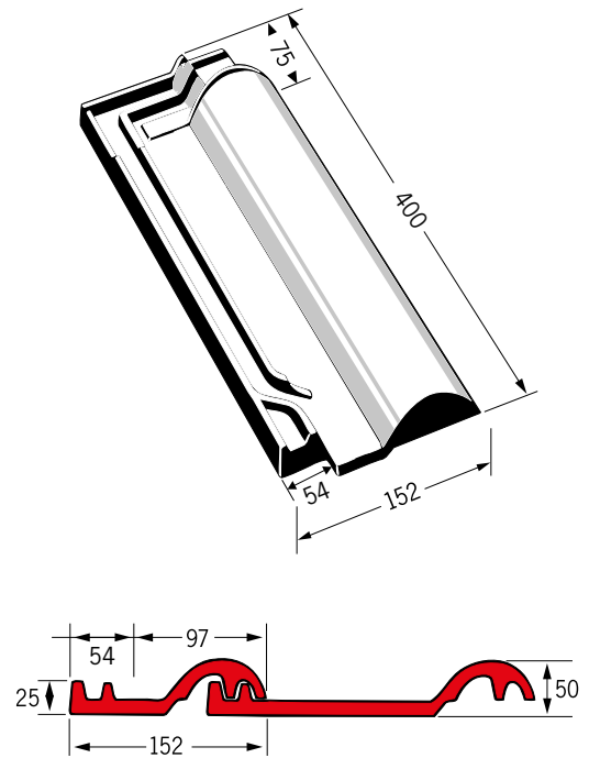
Garant halber Ziegel
