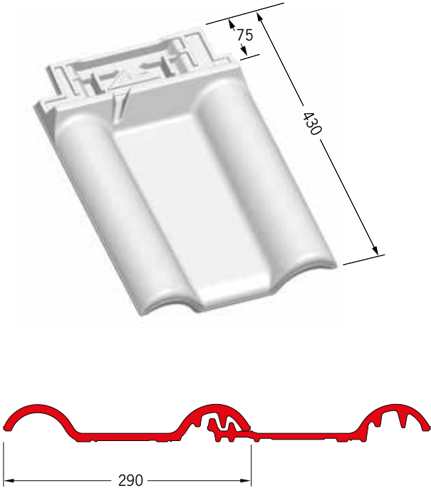
Opus® Firstanschluss Doppelwulst
