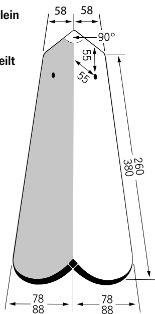
Biber Winkel klein, Rundschnitt
