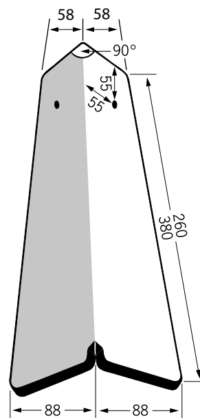
Biber Winkel klein, Geradschnitt
