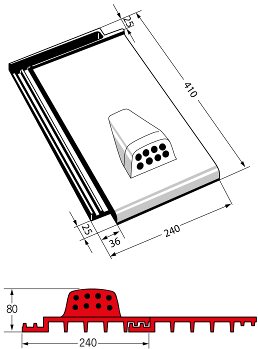
Piano Entlüftungsziegel
