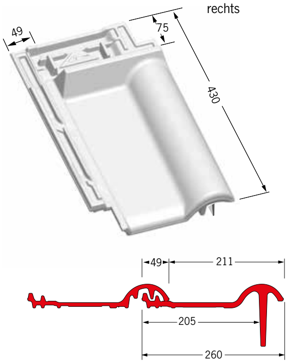
Opus® Firstanschluss Ortgangziegel
