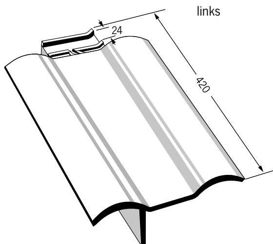
Ravensberger Ortgangziegel
