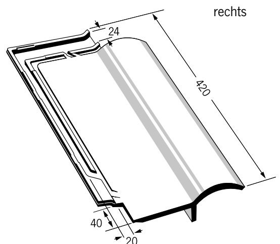
Ravensberger Ortgangziegel
