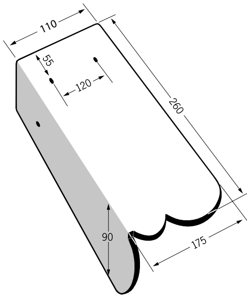
Biber Ortgang groß, links Rundschnitt geteilt
