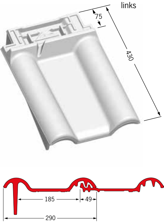
Opus® Firstanschluss Ortgangziegel
