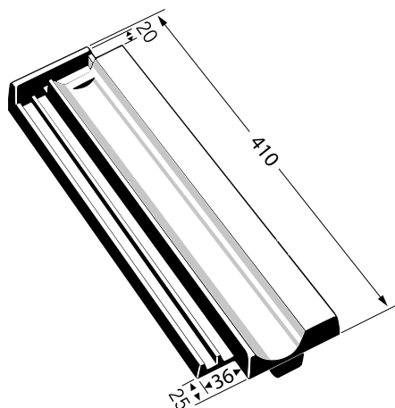
Dacapo halber Ziegel
