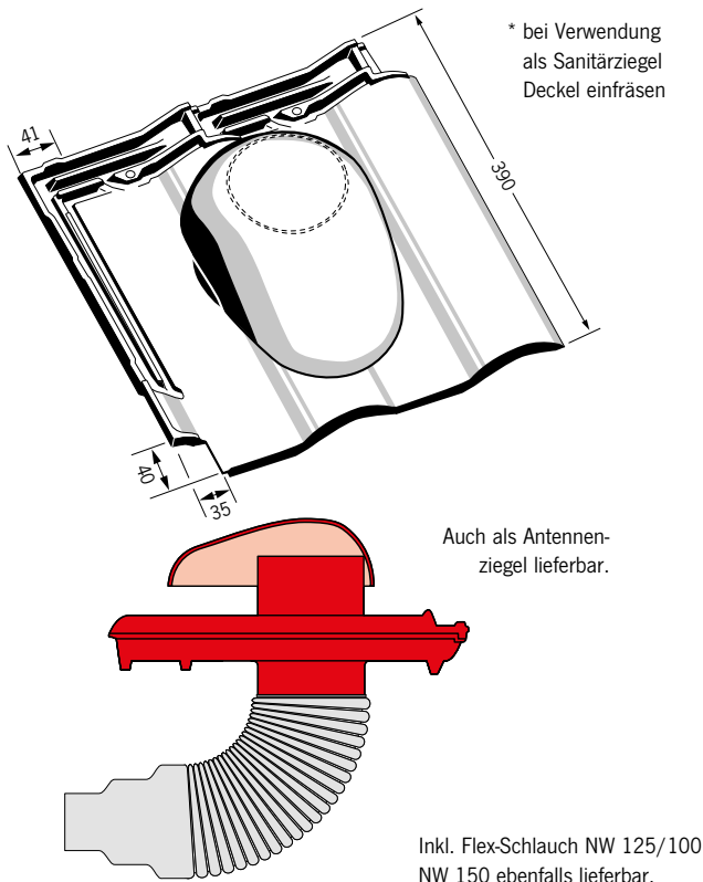
Tandem® Sanitär*-/Dunstrohrziegel
