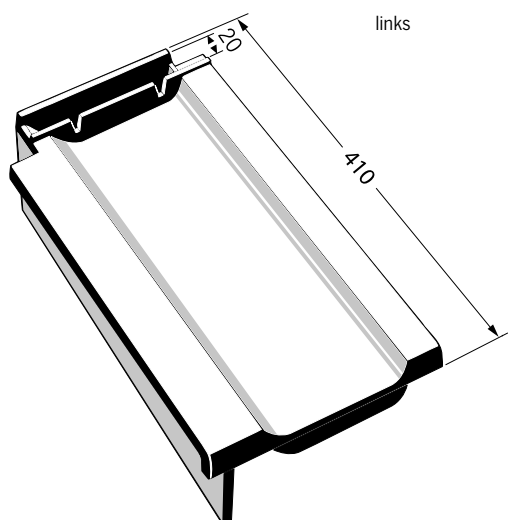
Dacapo Ortgangziegel
