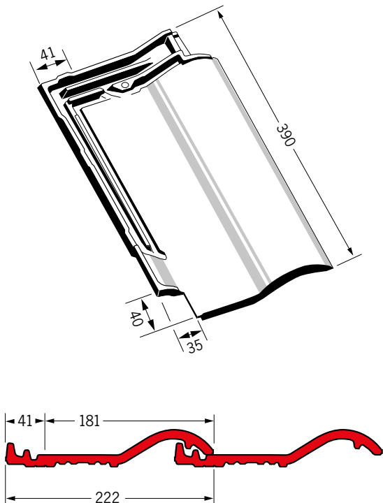
Tandem Junior®
