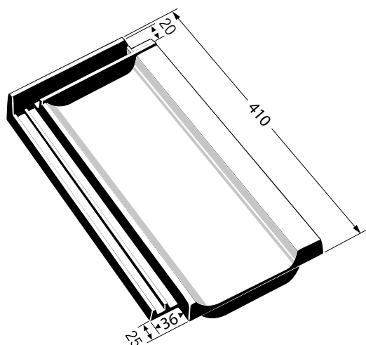
Dacapo Universaldachziegel
