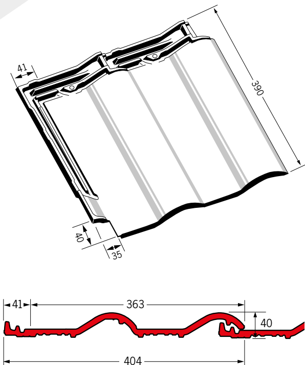
Tandem®
