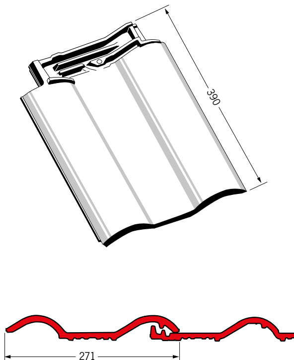
Tandem® Doppelwulstziegel
