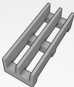
KABELKANAL K2 STD LIGHT
