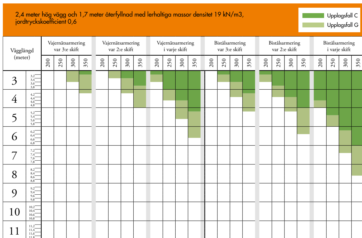
Diagram 2.2 Högsta tillåtna vägglängd mellan stödvägg på 2,4 m hög källarvägg återfylld med 1,7 m lerhaltiga massor vid olika armeringsintervall och blockstorlek.
