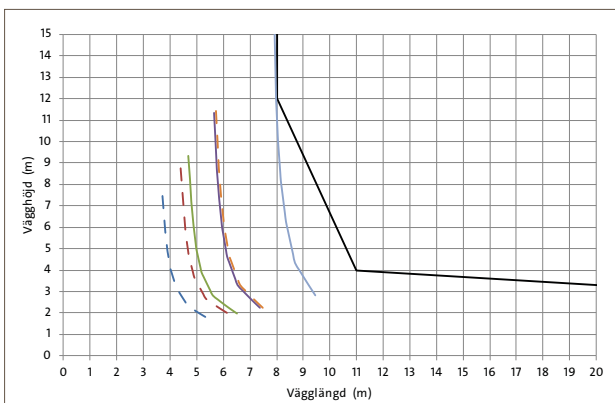
Diagram 3.5 Maximal väggstorlek för LECA block 200 med 1,2 kN/m 2 vindlast och upplag A.
