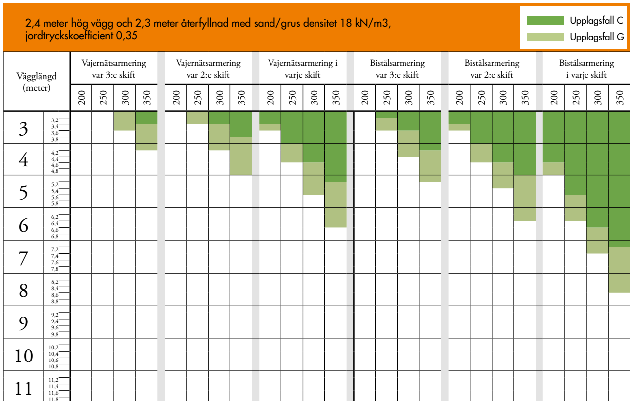
Diagram 2.4. Högsta tillåtna vägglängd mellan stödvägg på 2,4 m hög källarvägg återfylld med 2,3 m sand/grus vid olika armeringsintervall och blockstorlek.
