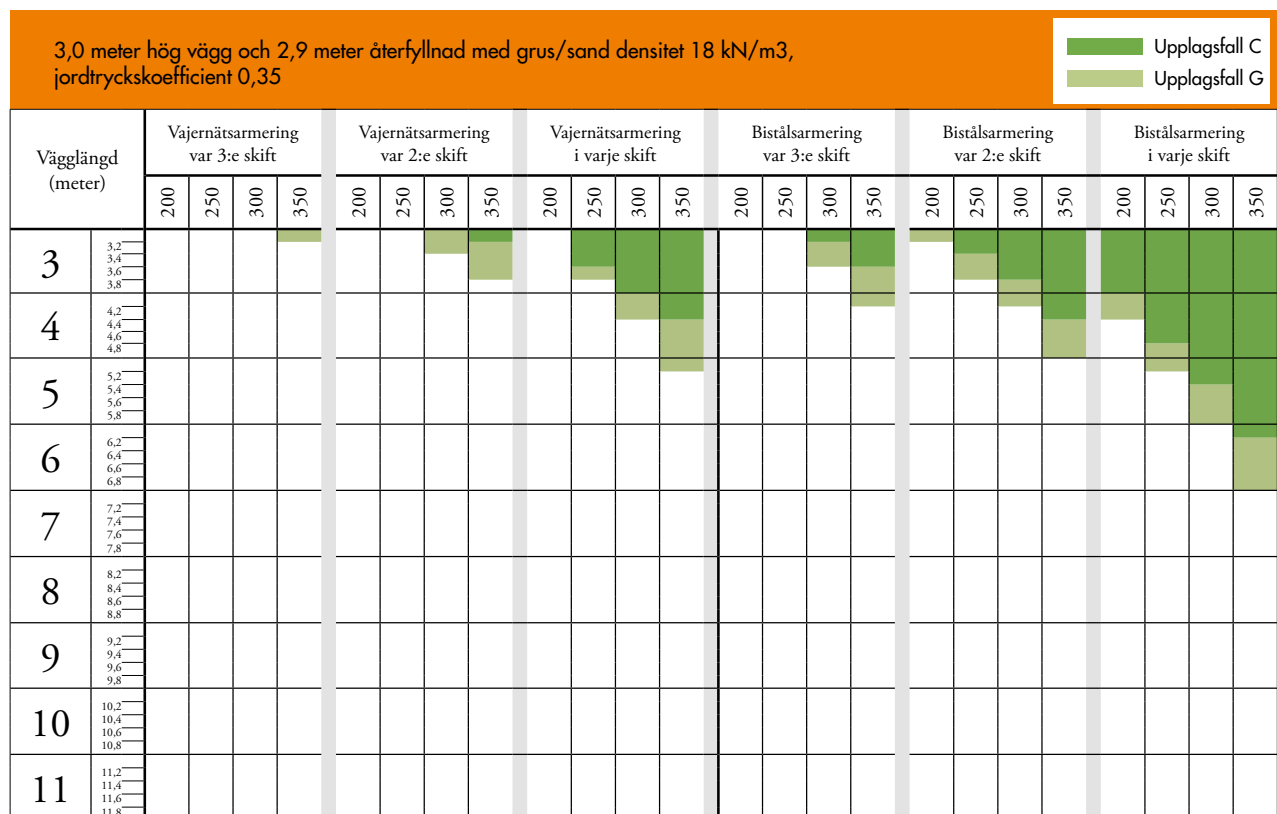
Diagram 2.7 Högsta tillåtna vägglängd mellan stödvägg på 3,0 m hög källarvägg återfylld med 2,9 m sand/grus vid olika armeringsintervall och blockstorlek.
