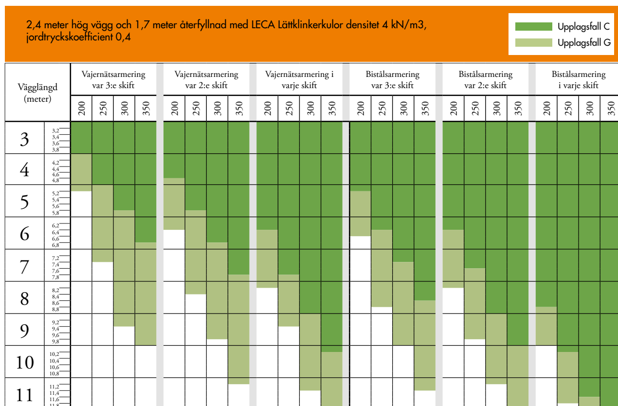
Diagram 2.3 Högsta tillåtna vägglängd mellan stödvägg på 2,4 m hög källarvägg återfylld med 1,7 m LECA Lättklinkerkulor vid olika armeringsintervall och blockstorlek.
