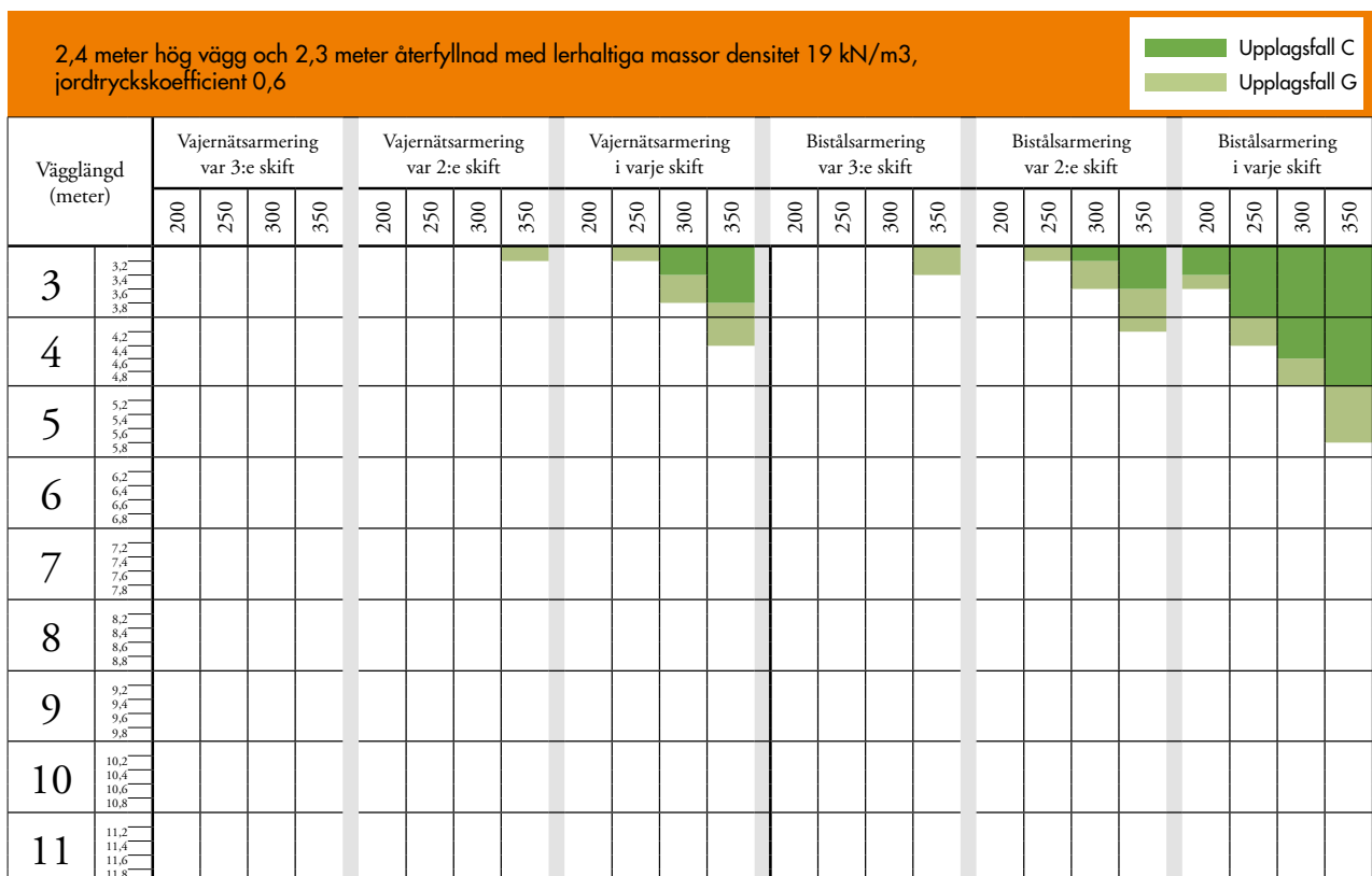
Diagram 2.5 Högsta tillåtna vägglängd mellan stödvägg på 2,4 m hög källarvägg återfylld med 2,3 m sand/grus vid olika armeringsintervall och blockstorlek.
