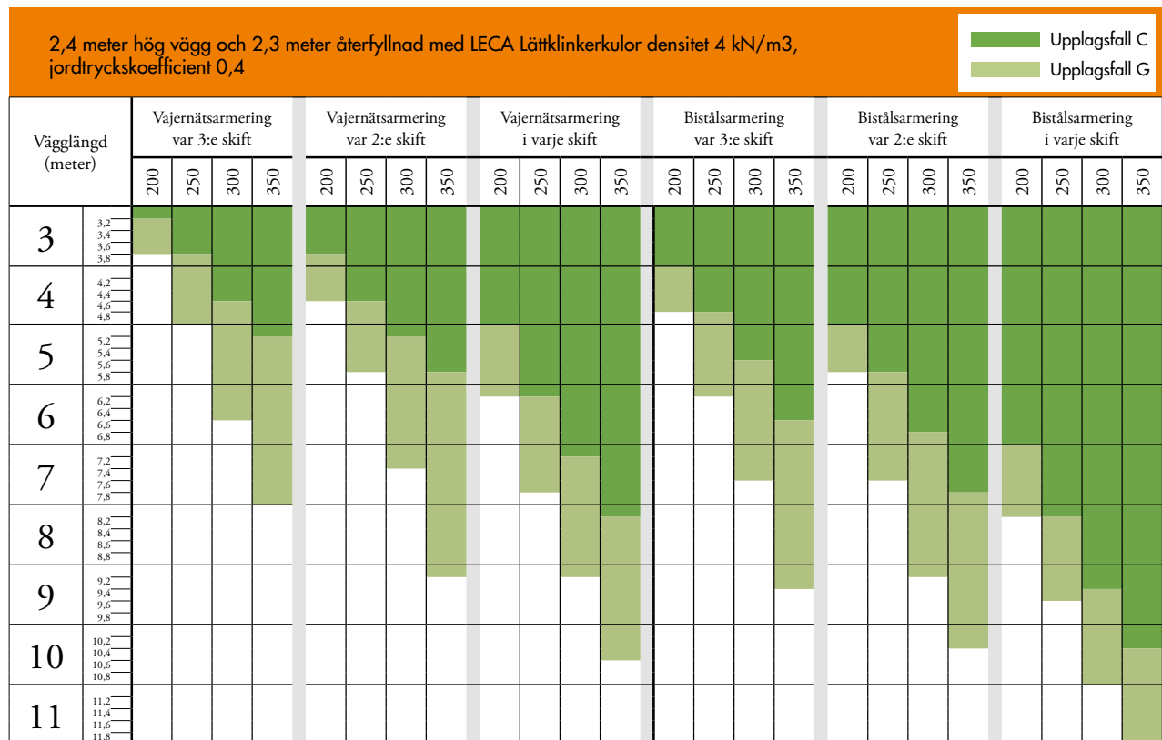
Diagram 2.6 Högsta tillåtna vägglängd mellan stödvägg på 2,4 m hög källarvägg återfylld med 2,3 m LECA Lättklinkerkulor vid olika armeringsintervall och blockstorlek.
