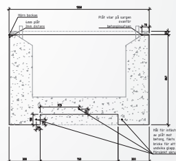
STÅLDETAJ - SEKTION A-A
