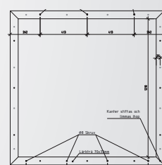
TRÄDETAJ - PLAN
