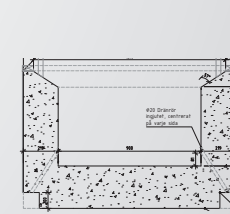
BETONGDETAJ - SEKTION A-A
