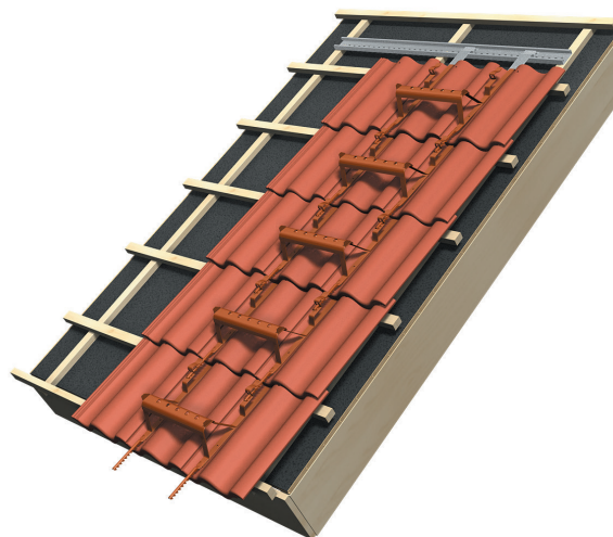
Kopplade taksteg monterade på tak
