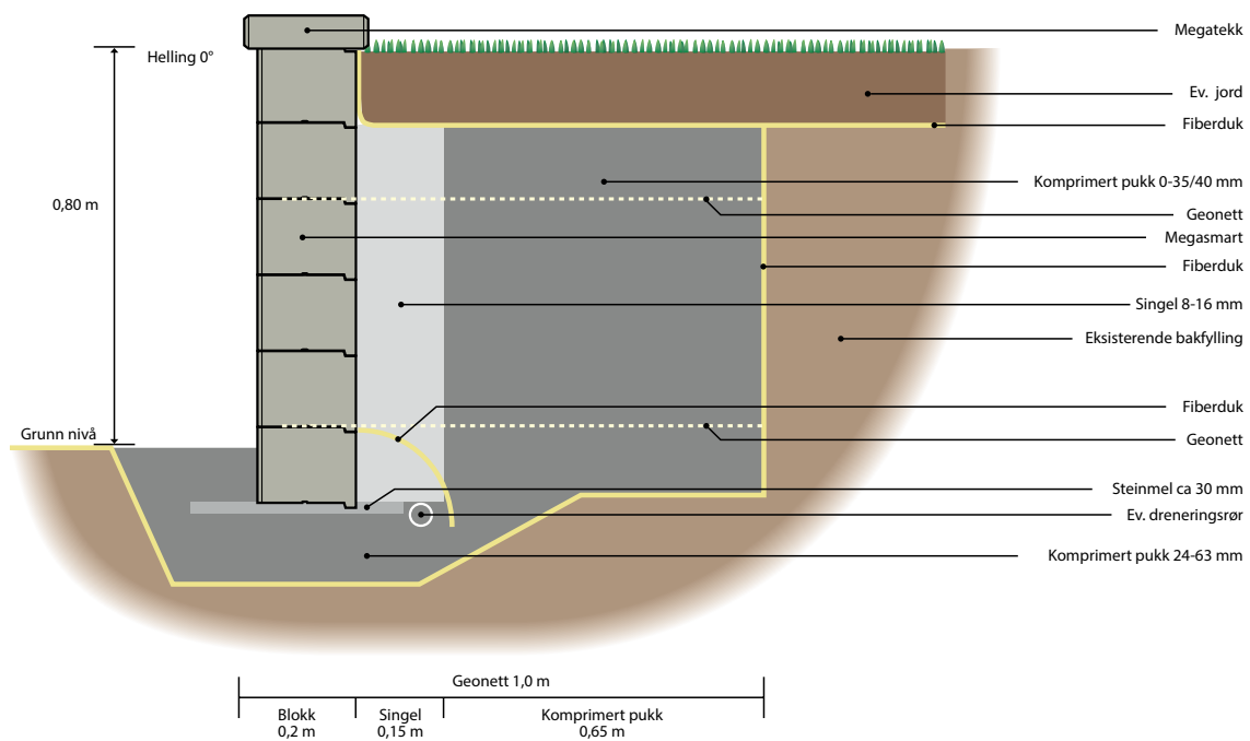
Bilde 4. Snittegning loddrett støttemur med geonett, opp til 0,8 m.
