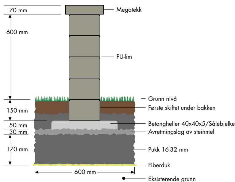
Bilde 1. Snittegning Megalock, 4 skift over bakken
