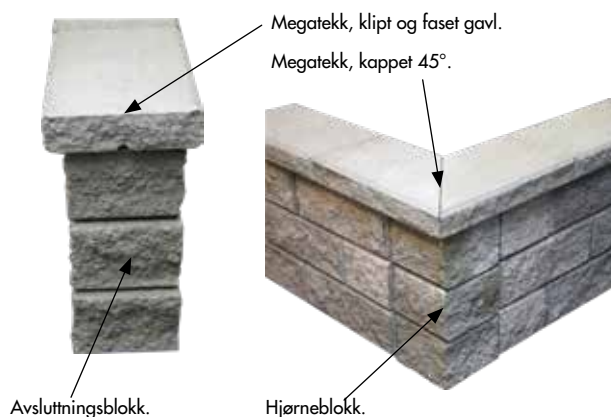
Bilde 2. Megaloc Avslutningsblokk.
