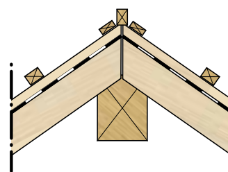
Qube/Vinklet møne
