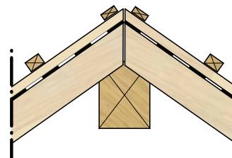
Qube/Vinklet møne
