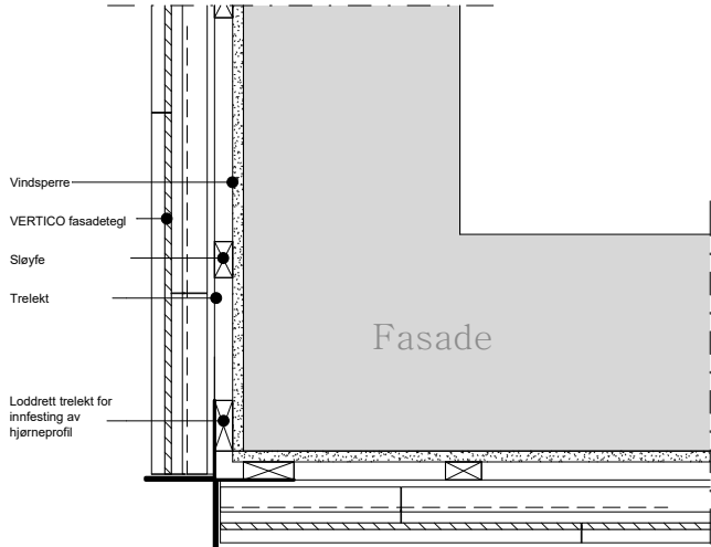
Lokalt tilpasset hjørnebeslag
