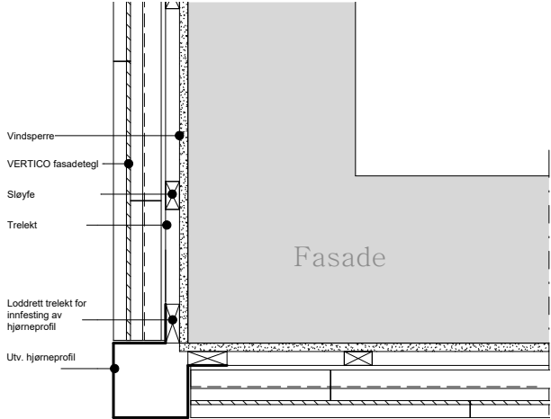
Vertico utvendig hjørneprofil
