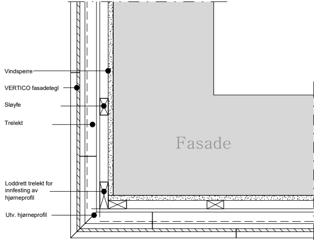
Vertico utvendig hjørne i tegl
