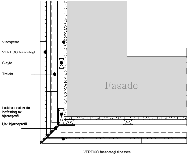
Vertico utvendig hjørneprofil - skrå
