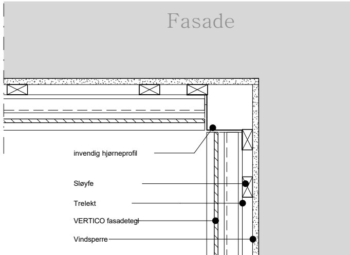
Vertico innvendig hjørneprofil
