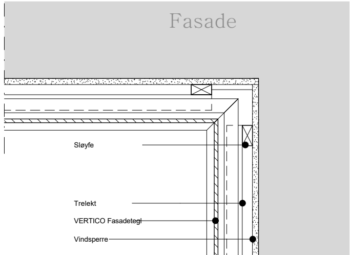
Vertico innvendig hjørne i tegl
