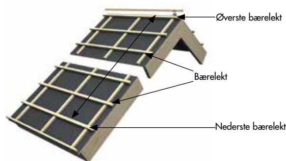
Figur 5. Avstanden mellom øvre og nedre bærelekt brukes ved utregningen av lekteavstand.
