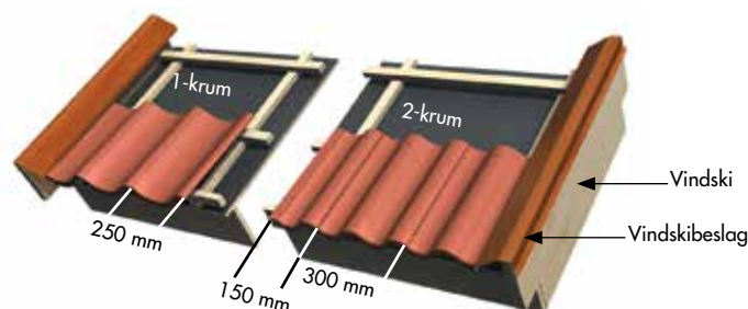
Figur 8. Del opp taket i antall takstein. Husk at siste takstein ut mot venstre gavel bygger 280 mm for enkelkrum.
