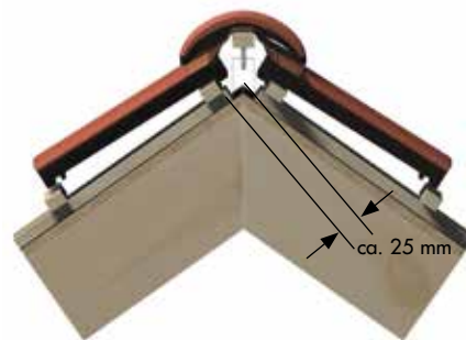
Figur 4. Den øverste bærelekten festes ca. 15-40 mm mm fra takspissen
