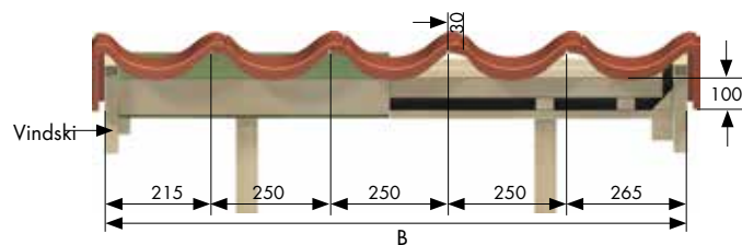
Figur 21. Gavlsteininndeling for enkelkrum. Separat tabell for målinndeling av tak finnes på vår hjemmeside.
