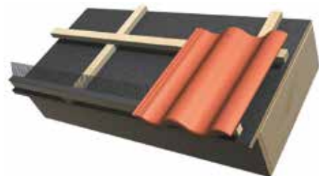
Figur 3. Fuglebåndet monteres på takfotslekten. (Takfotslekten skal være 10 mm høyere enn bærelekten.) Ved bruk av ventilert fuglebånd har dette en byggehøyde på 25 mm.
