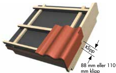
Figur 20. Benders gavlstein gir meget god tetting samtidig som man slipper vedlikeholdsarbeidet som du får på vindski og israft i trematerialet. Det skal brukes 110 mm ved lekteravstand 310-335 mm og 88 mm brukes ved lekteravstand 336-375 mm.
