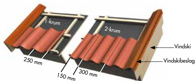
Figur 8. Del opp taket i antall takstein. Husk at siste takstein ut mot venstre gavel bygger 280 mm for enkelkrum.
