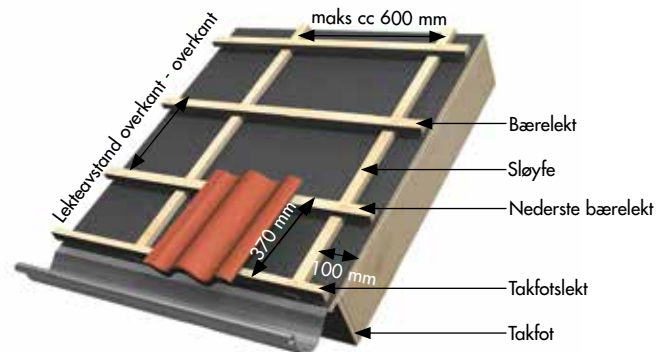
Figur 2. Lekteavstand måles fra overkant til overkant. Merk at målet på første bærelekt er fra nedkant takfot til overkant første bærelekt. Dette målet er 370 mm. Hvis takfoten avsluttes vinkelrett mot takfallet og det ikke benyttes takfotbeslag, anbefaler vi at målet fra nedkant takfot til overkant første bærelekt er 340 mm.
