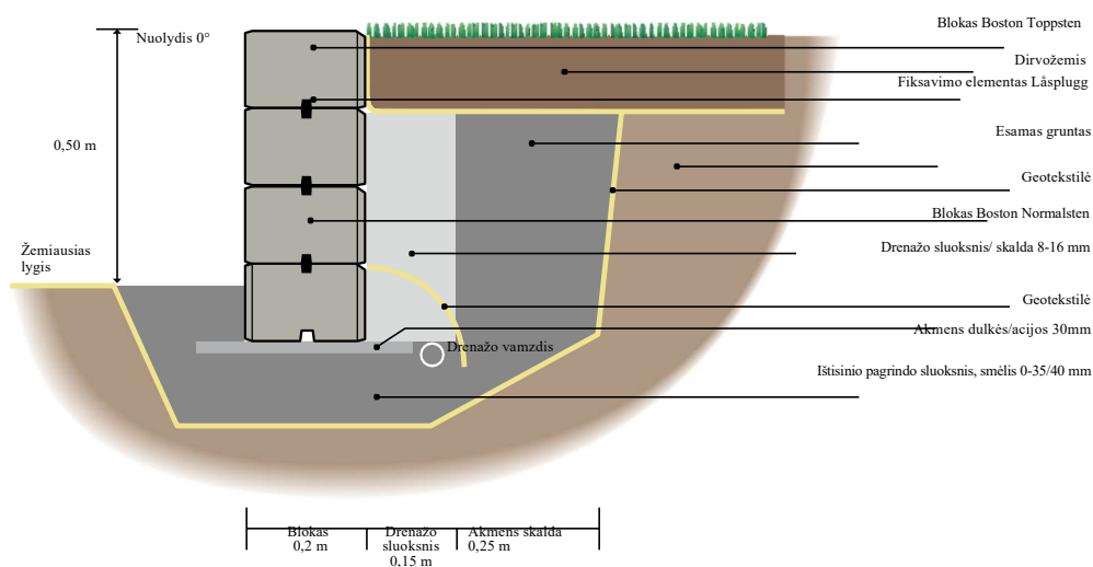
Pav.1 Atraminė siena iki 0,5 m aukščio.
