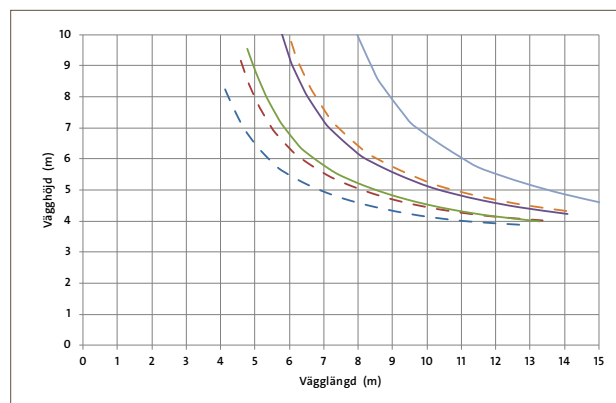
Diagram 3.33 Maximal väggstorlek för LECA block 350 med 1,2 kN/m 2 vindlast och upplag K.
