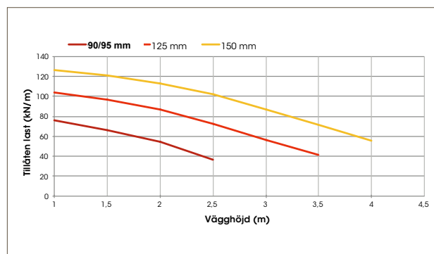
Diagram 4.1 Vertikal last på innervägg.
