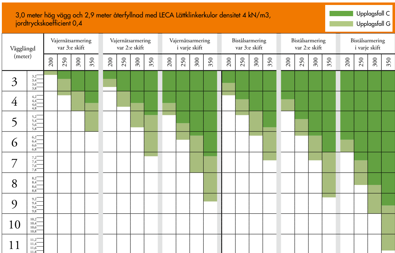
Diagram 2.9 Högsta tillåtna vägglängd mellan stödväggar på 3,0 m hög källarvägg återfylld med 2,9 m LECA Lättklinkerkulor vid olika armeringsintervall och blockstorlek.
