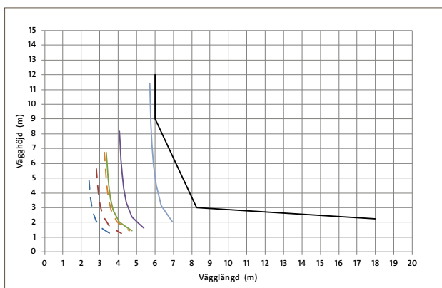
Diagram 3.4 Maximal väggstorlek för LECA block 150 med 1,2 kN/m 2 vindlast och upplag A.
