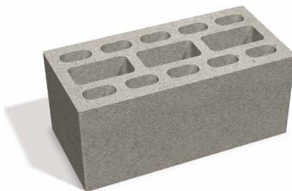
Bender Betonghålsten
