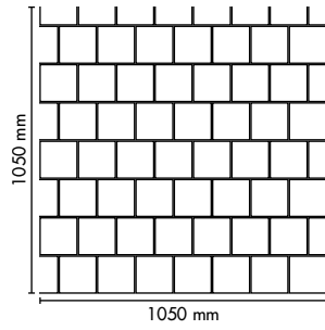
1/2 förband
