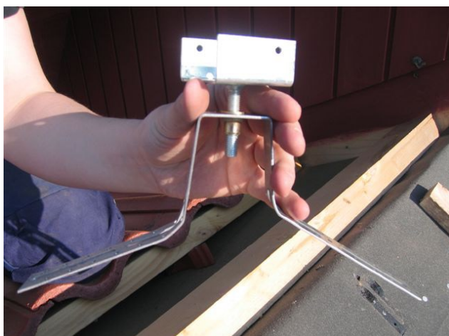
Monteringsbild 2. Böcka U-benen så du erhåller rätt höjd, finjustering kan du göra senare. Tänk på att U-benen skall ligga ovan bärläkt på lätt undertak och ovan ströläkt vid traditionellt tak (råspont).
