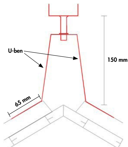
Bild 3. Vid högsta montering av nockbrädes hållare, finns en justermån på 125 - 150 mm. Knäckmättet är på bilden 65 mm, vilket är minimum knäckmätt för tillräcklig infästning.
