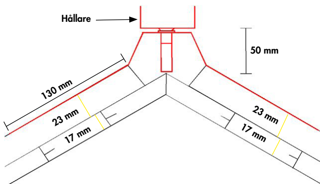
Bild 2. Vid lägsta montering av nockbrädes hållare, finns en justermån på 50 - 75 mm. Knäckmättet är på bilden 130 mm, vilket är max knäckmätt. Det finns då plats mellan U-benens topp och nockspetsen för lägsta justering, 50 mm.
