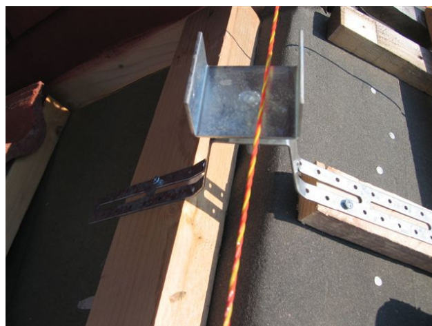
Monteringsbild 4. Montera ett snöre i centrum av de båda nockhållarna som placerats på taket. Montera dit resterande nockhållare som nu får rätt höjd och även görnocken absolut rak. Bilden visar höger sida råspontmontage, vänster sida lätt undertak.
